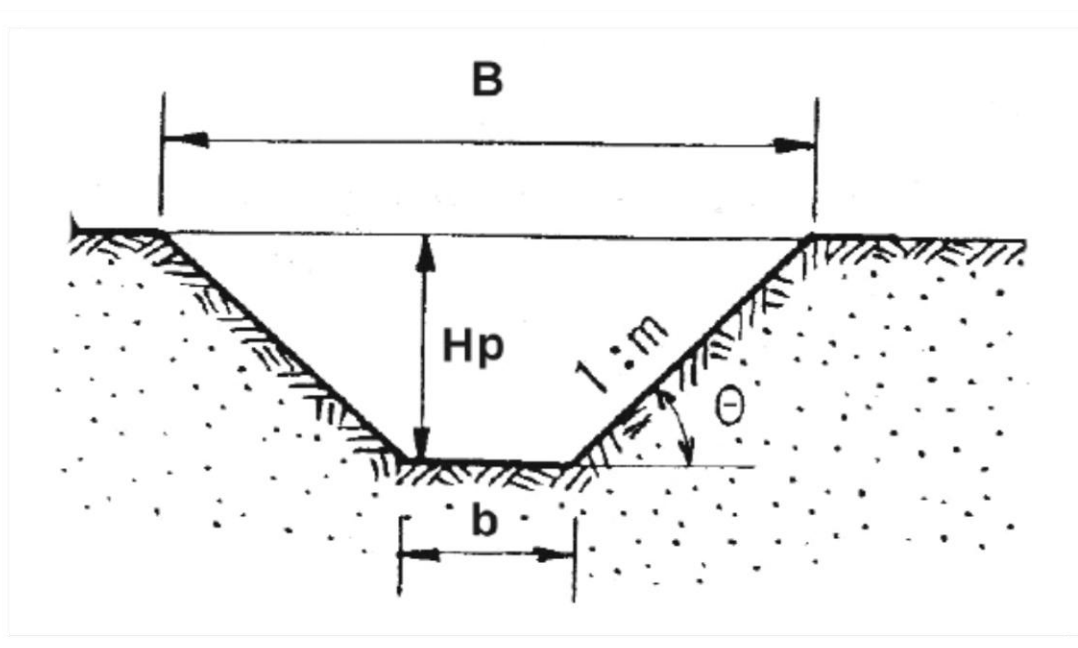
Слика 16: Изглед профила канала
