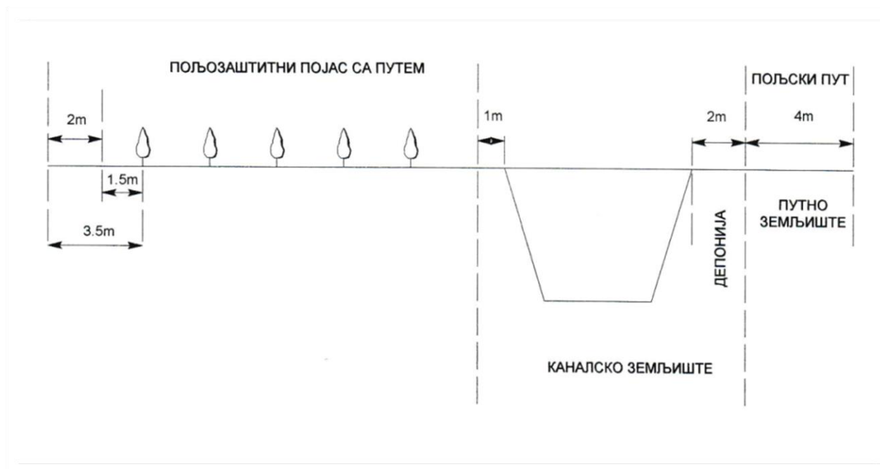
Слика 17: Пример профила пољозаштитног појаса са пољским путем и каналом
