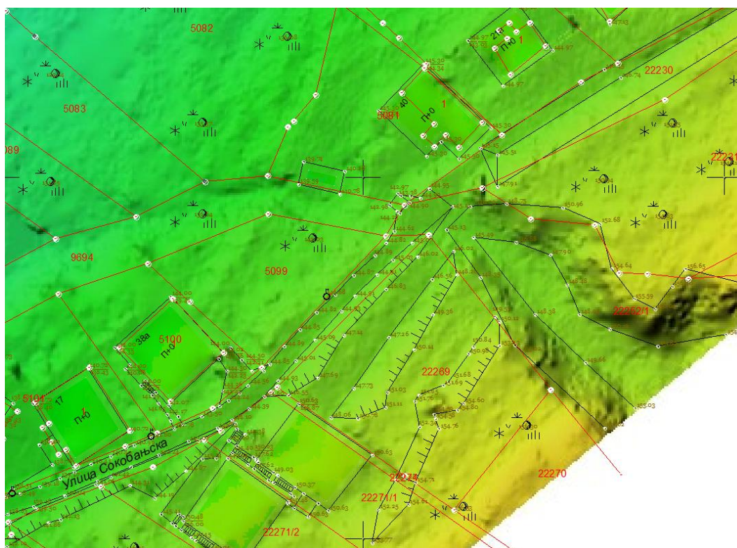
Слика 11: Интегрисана геореференцирана слика ДМТ
