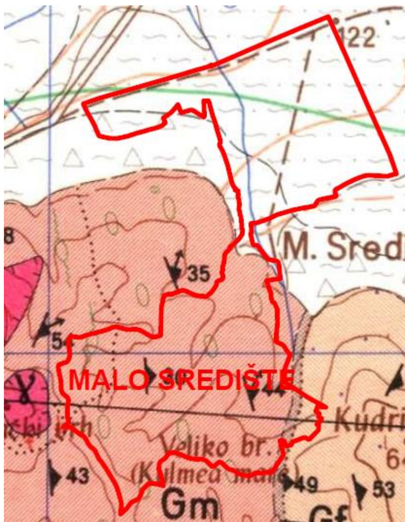
Слика 4: Геолошка карта КО Вршац
