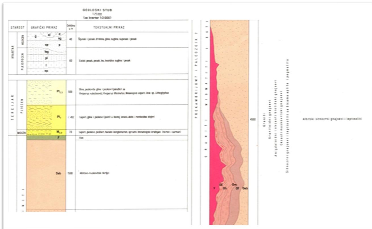
Слика 6: Геолошки стуб КО Вршац
