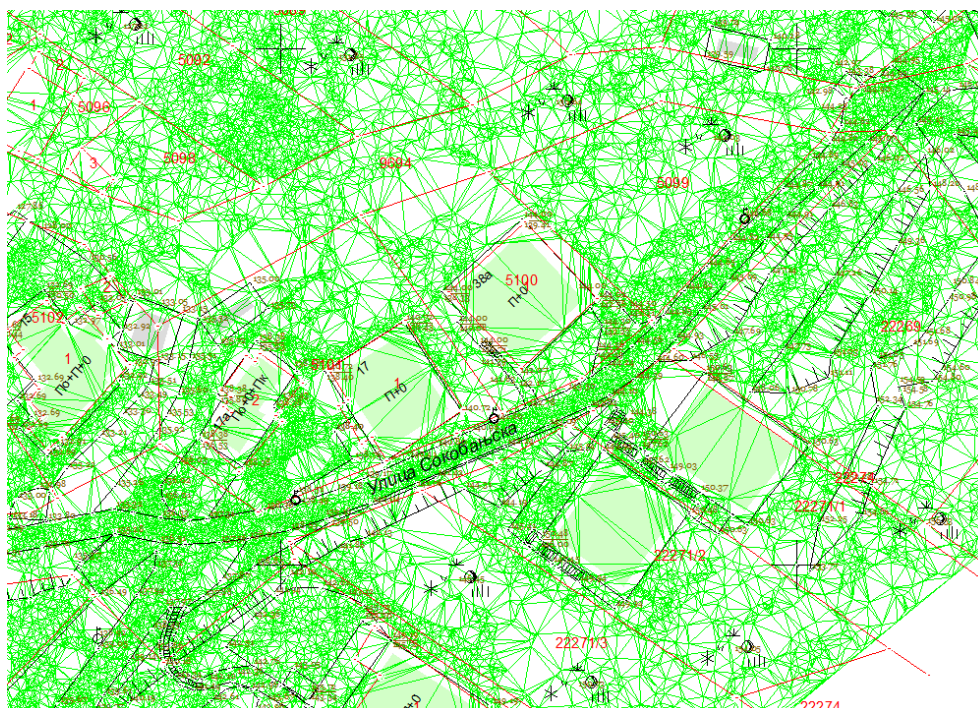
Слика 10: Приказ ДМТ као мреже троуглова (ТИН) израђен на основу 3Д облака тачака површи терена
